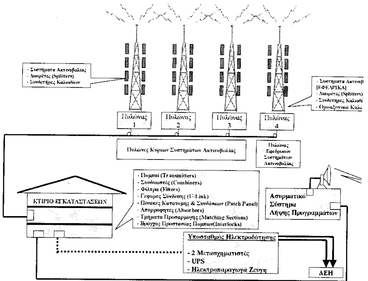
Σχήμα 2.1: Αρχιτεκτονική Πάρκου Κεραιών
