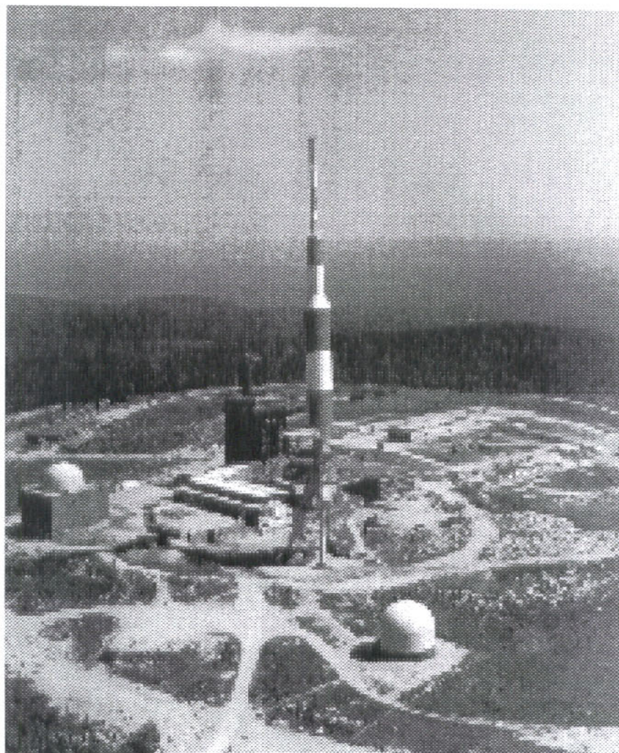
Σχήμα 7.9: Εγκατάσταση Brocken
