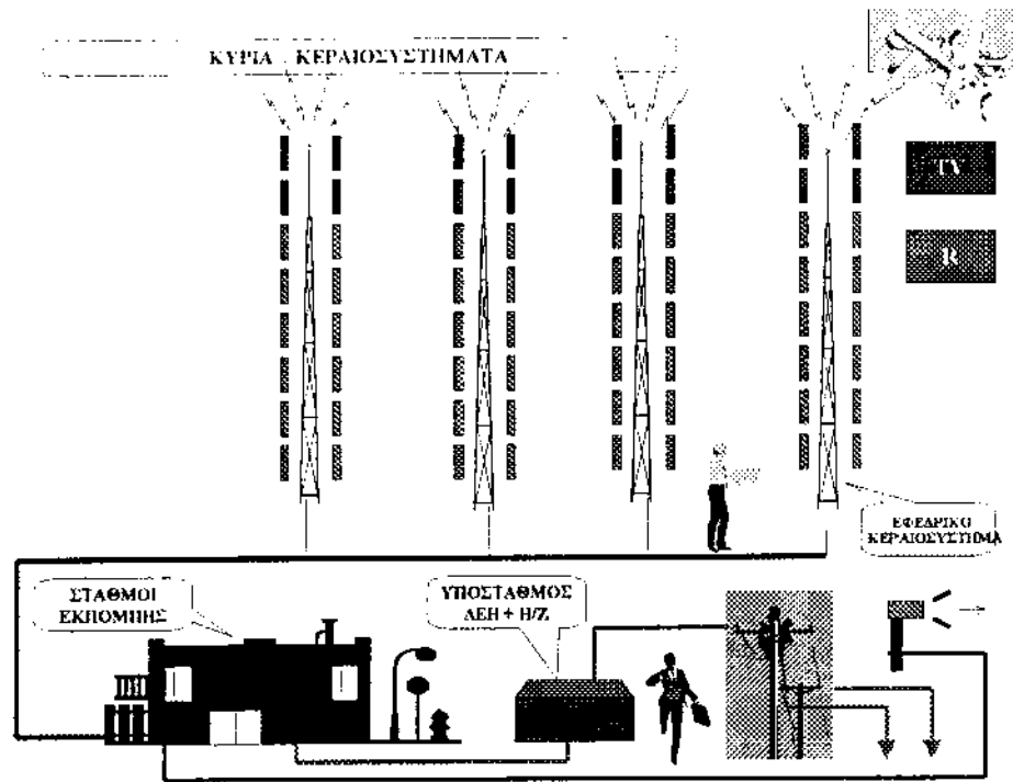
Σχήμα 2.2: Περιγραφή του εξοπλισμού του Πάρκου Κεραιών
