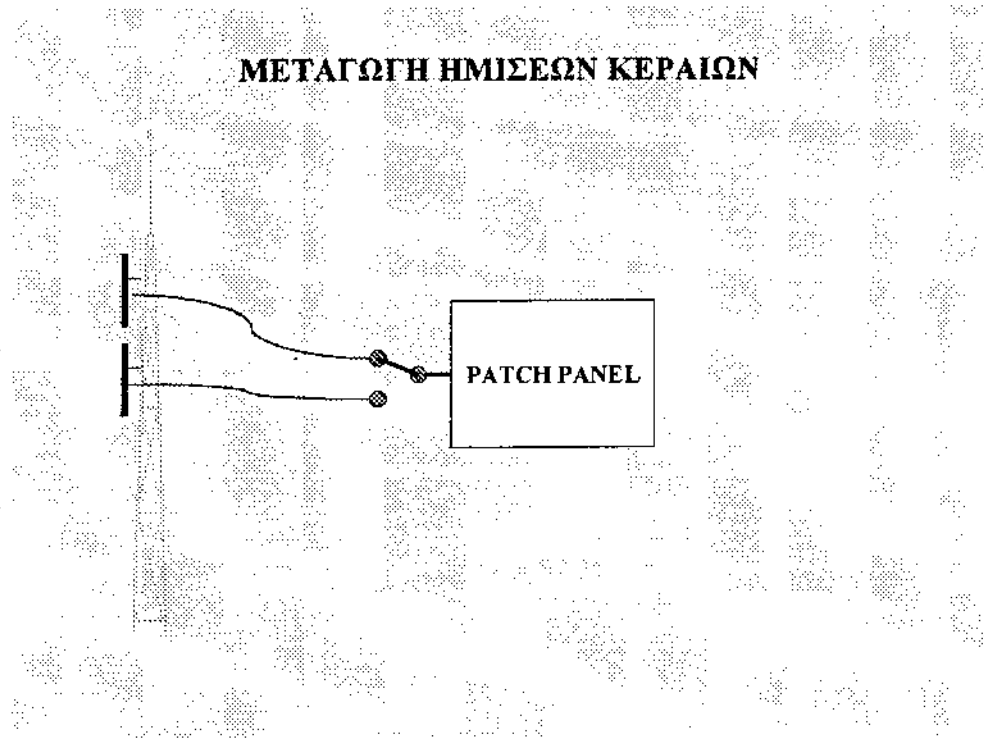
Σχήμα 2.6: Μεταγωγή Ημίσεων Κεραιών
