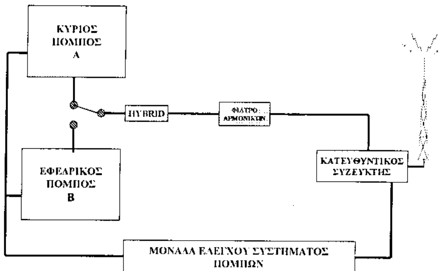
Σχήμα 2.5: Μεταγωγή Πομπών
