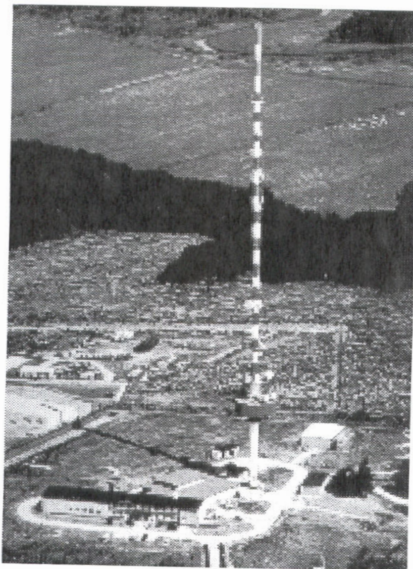
Σχήμα 7.12: Εγκατάσταση Marlow
