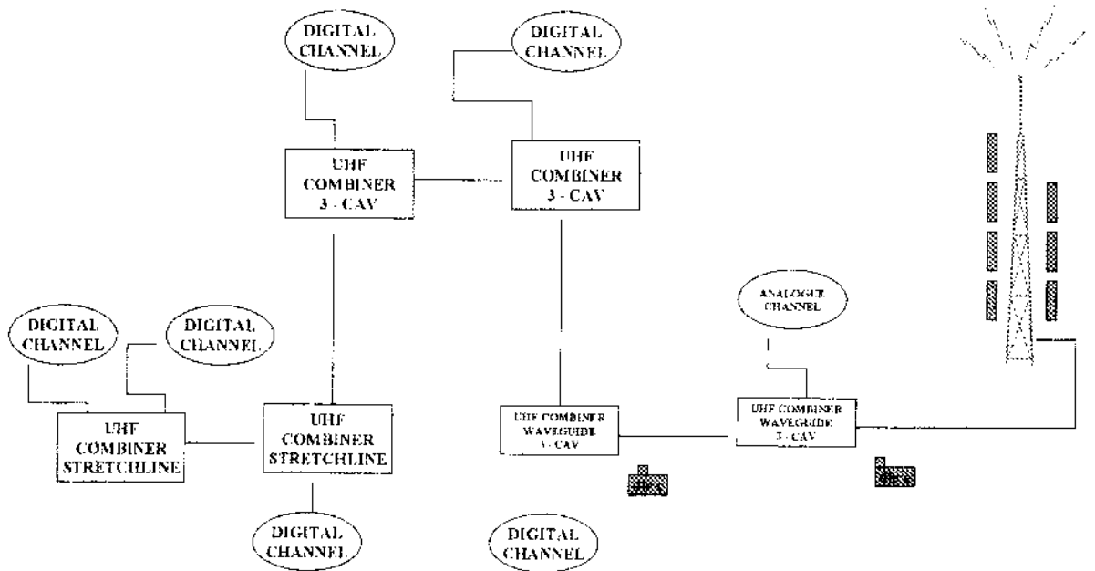
Σχήμα 7.6: Μπλοκ διάγραμμα Πάρκου Κερατών Craigkelly, NTL
