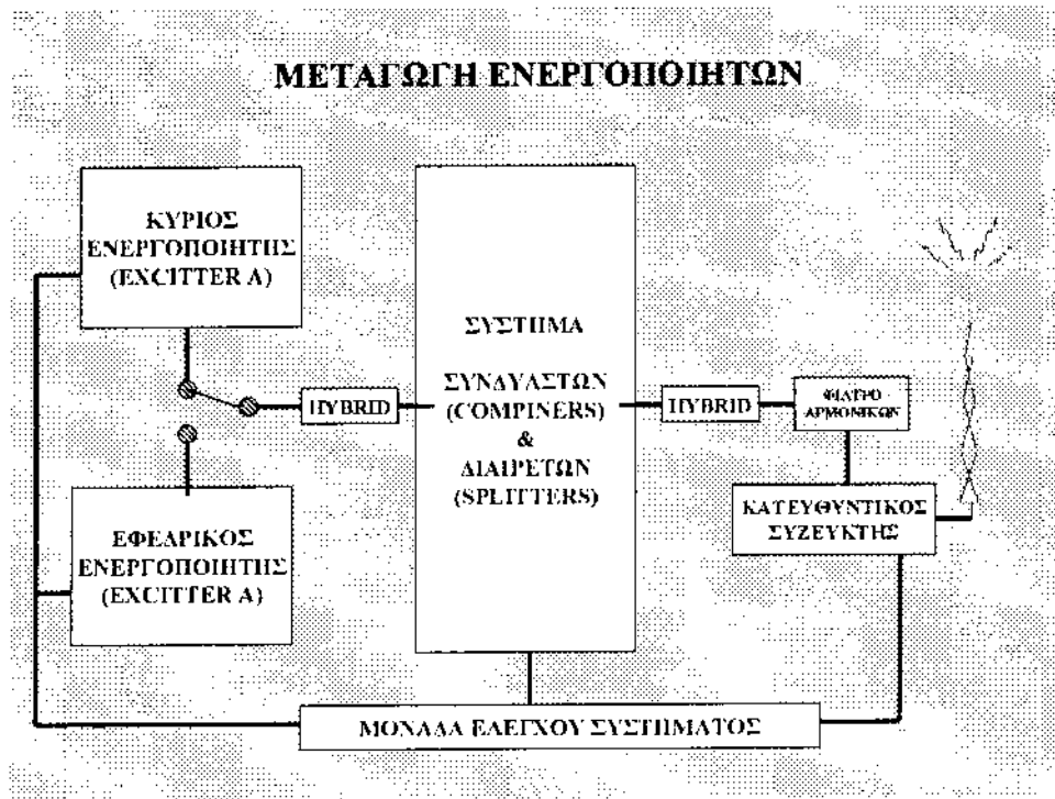
Σχήμα 2.4: Μεταγωγή Ενεργοποιητών
