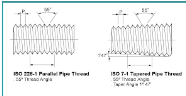
Διαφορά παράλληλου και κωνικού αρσενικού σπειρώματος
