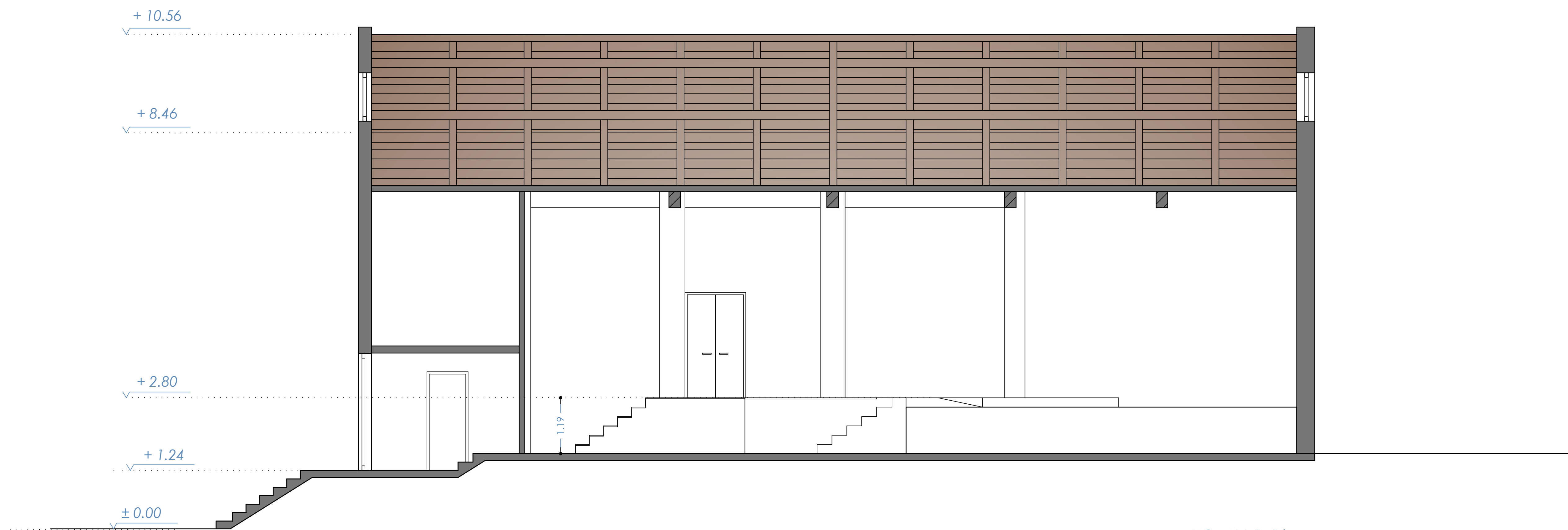
ΤΟΜΗ Β-Β'
